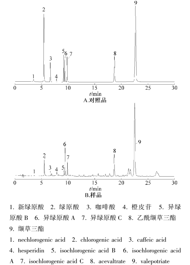
图 1 各成分 UPLC 色谱图
